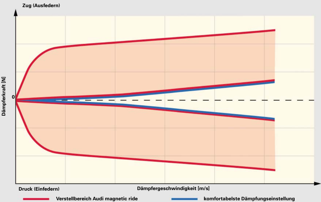
Dämpferkraftkennfeld Audi magnetic ride
