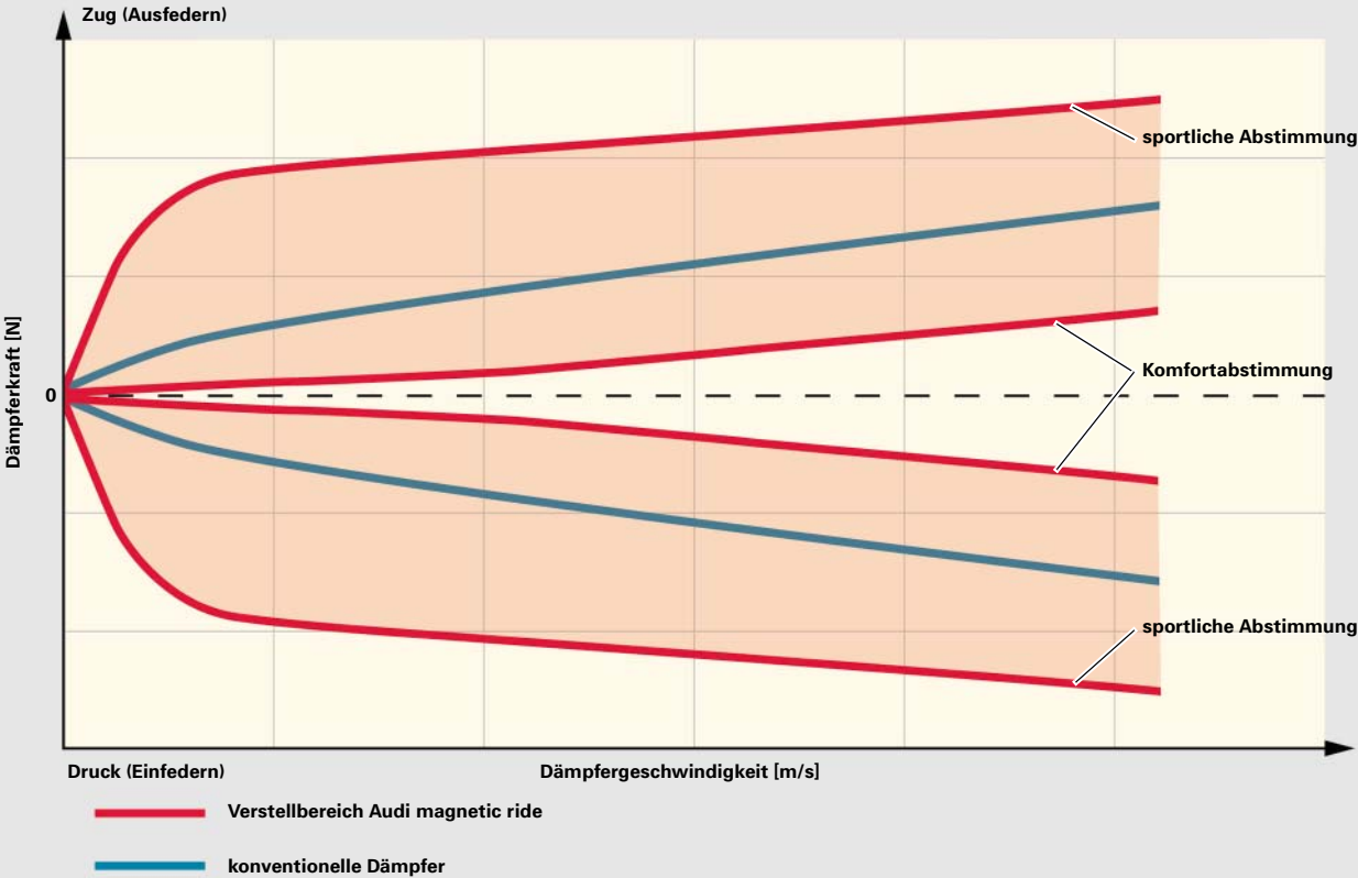
Vergleich der Dämpferkraftkennfelder Audi magnetic ride zu konventionellen Dämpfern
